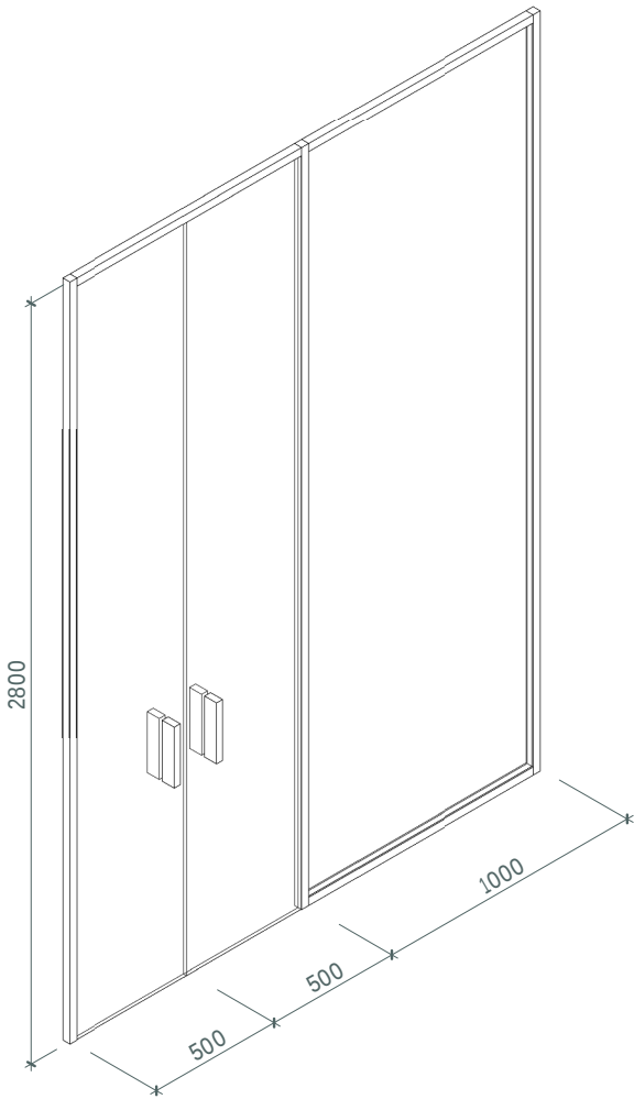
T2 (Скляна перегородка в гардероб)
