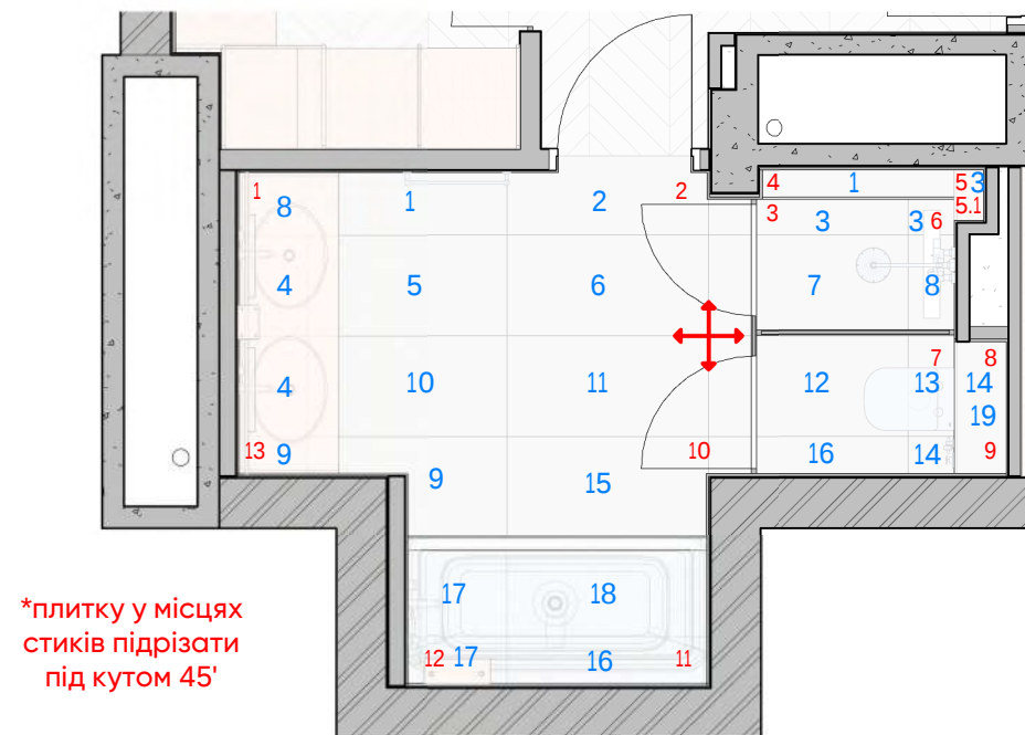
План (Мастер санвузол)
