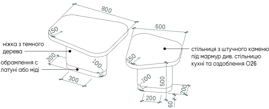
аксонометрія F17.1, F17.2
