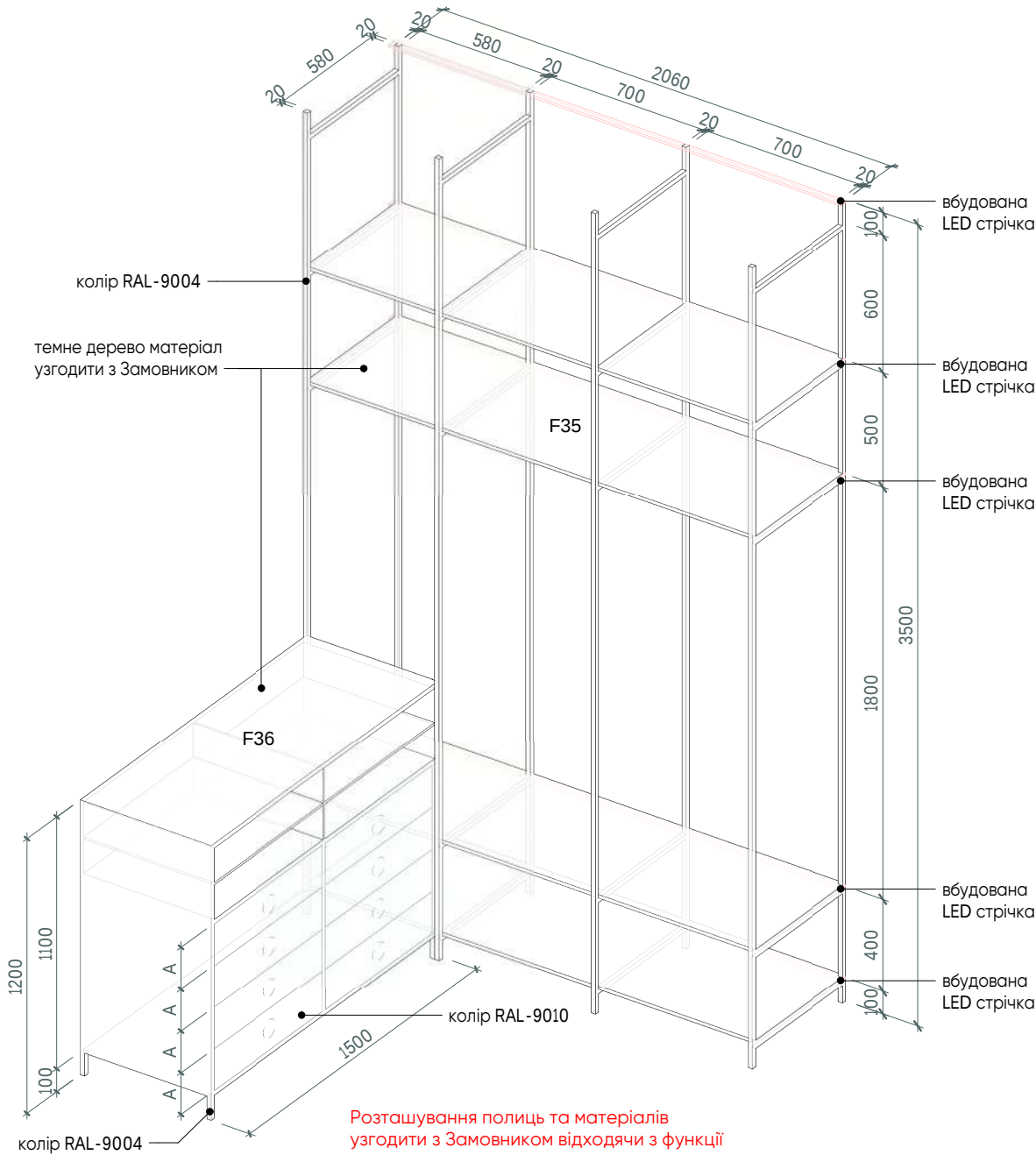
аксонометрія F35, F36
